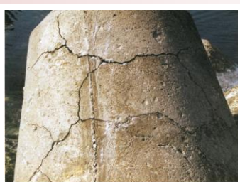
アルカリ骨材反応によるひび割れ
